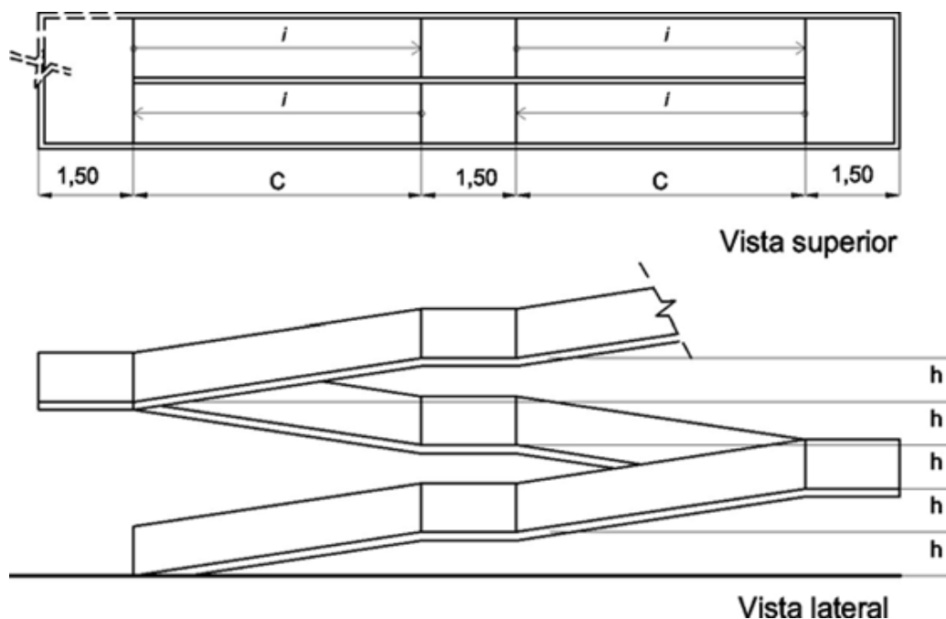
FIGURA 64 – Demonstração de uma vista superior e lateral de um esquema de Rampas.
