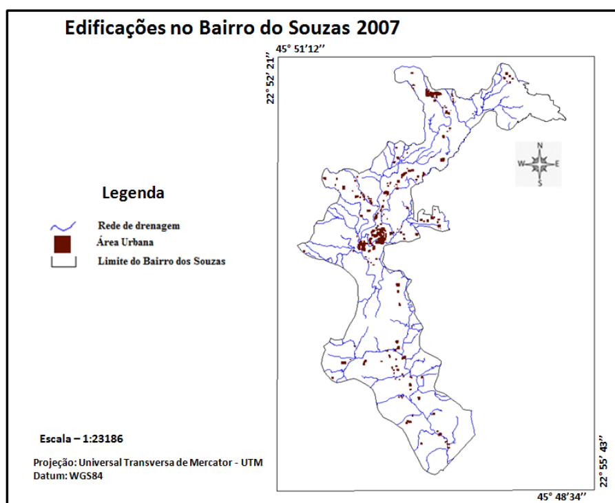
Figura 29: Edificações para o Bairro dos Souzas para o ano de 2007 no município de Monteiro Lobato.
