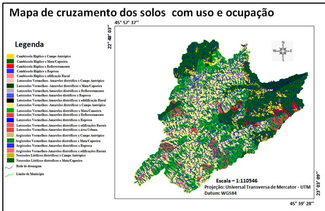
Figura 31: Distribuição do uso e ocupação do solo em cada unidade presente no município de Monteiro Lobato.
