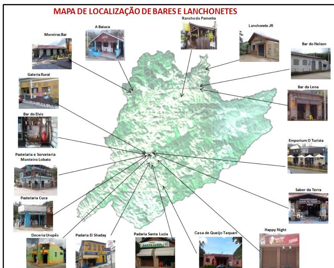
Figura 04: Mapa de localização de Bares e Lanchonetes
