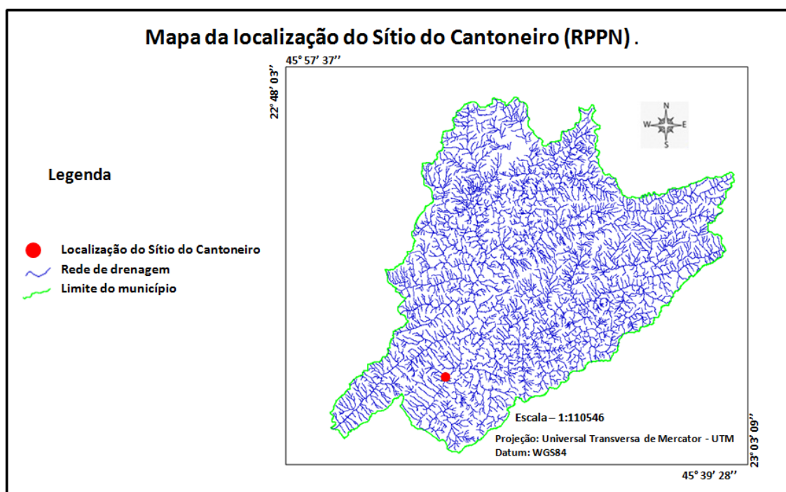
Figura 19: Localização do Sítio do Cantoneiro (RPPN) em Monteiro Lobato. Fonte: Bertoldo (2019)
