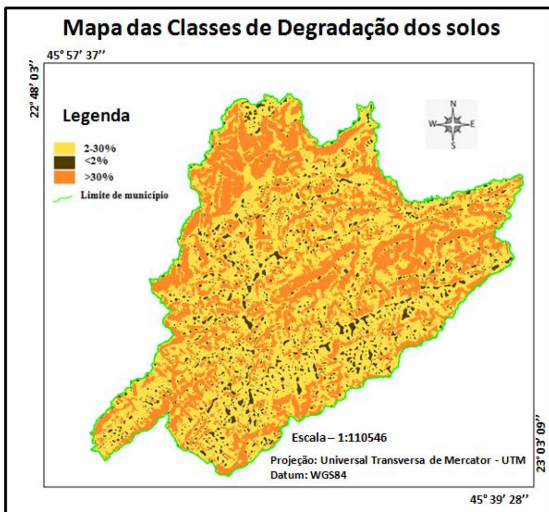
Figura 16: Distribuição territorial das classes de declividade para análise do potencial de degradação do solo no município de Monteiro Lobato.
