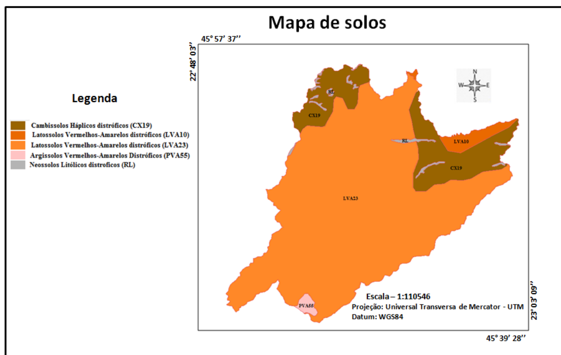
Figura 13: Distribuição das unidades de solos para Monteiro Lobato. Fonte: Oliveira (1999) (adaptado)
