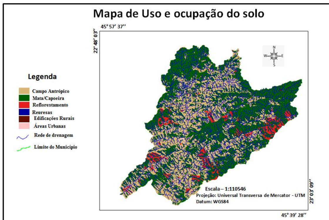
Figura 12: Mapa de uso e ocupação do solo de Monteiro Lobato.
