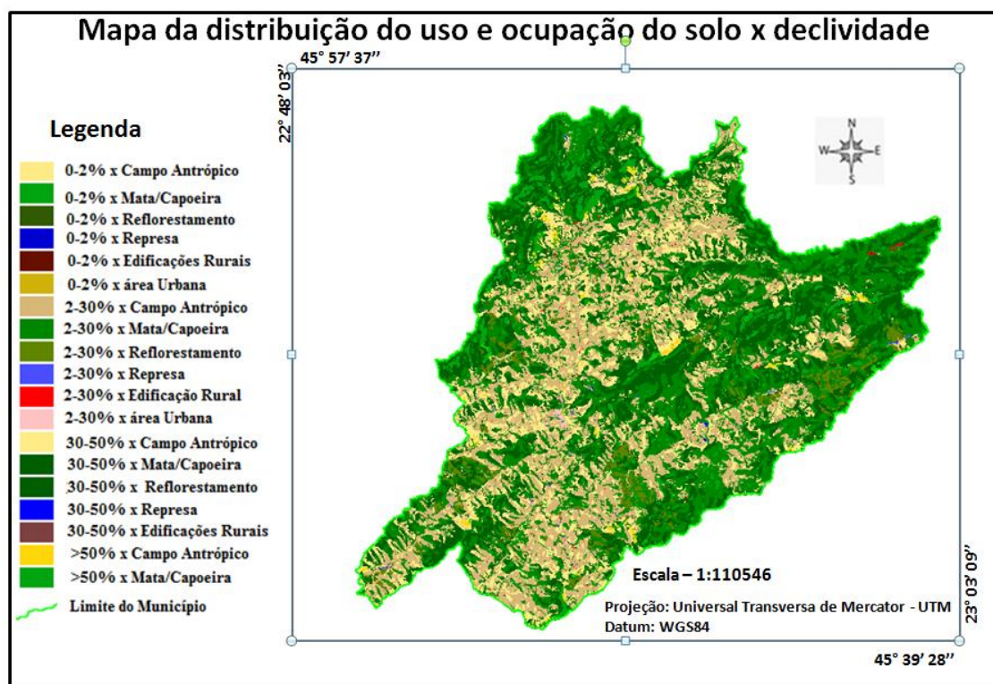
Figura 32: Distribuição das classes de uso e ocupação do solo de acordo com a distribuição da declividade analisada no município de Monteiro Lobato SP.
