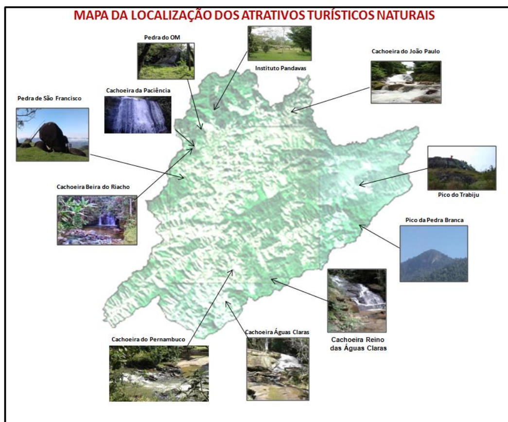
Figura 06: Mapa de localização dos Atrativos Naturais
