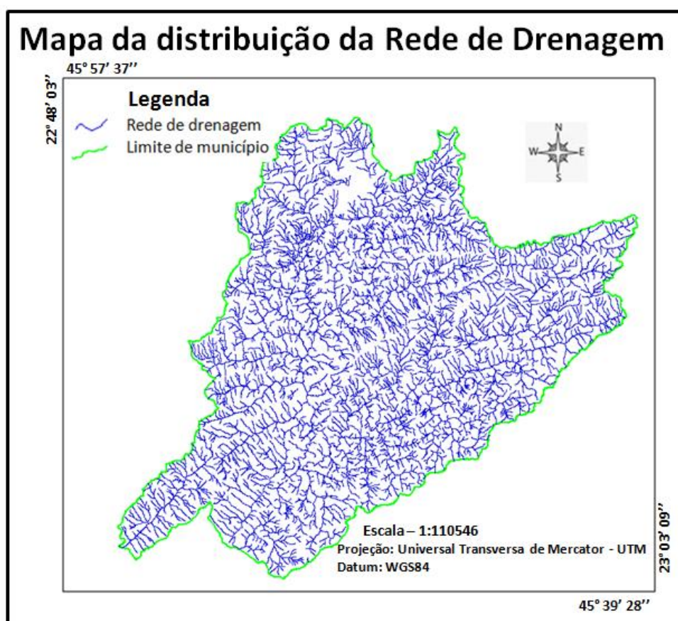
Figura 15: Distribuição da rede de drenagem no município de Monteiro Lobato.
