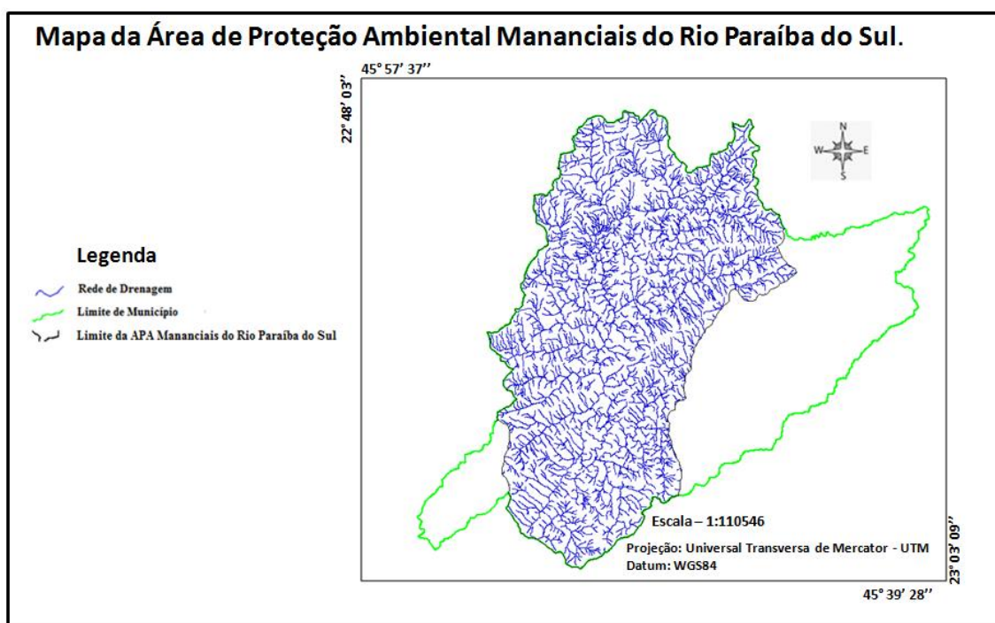
Figura 17: Localização da Área de Proteção Ambiental – APA Mananciais do Rio Paraíba do Sul no município de Monteiro Lobato.
