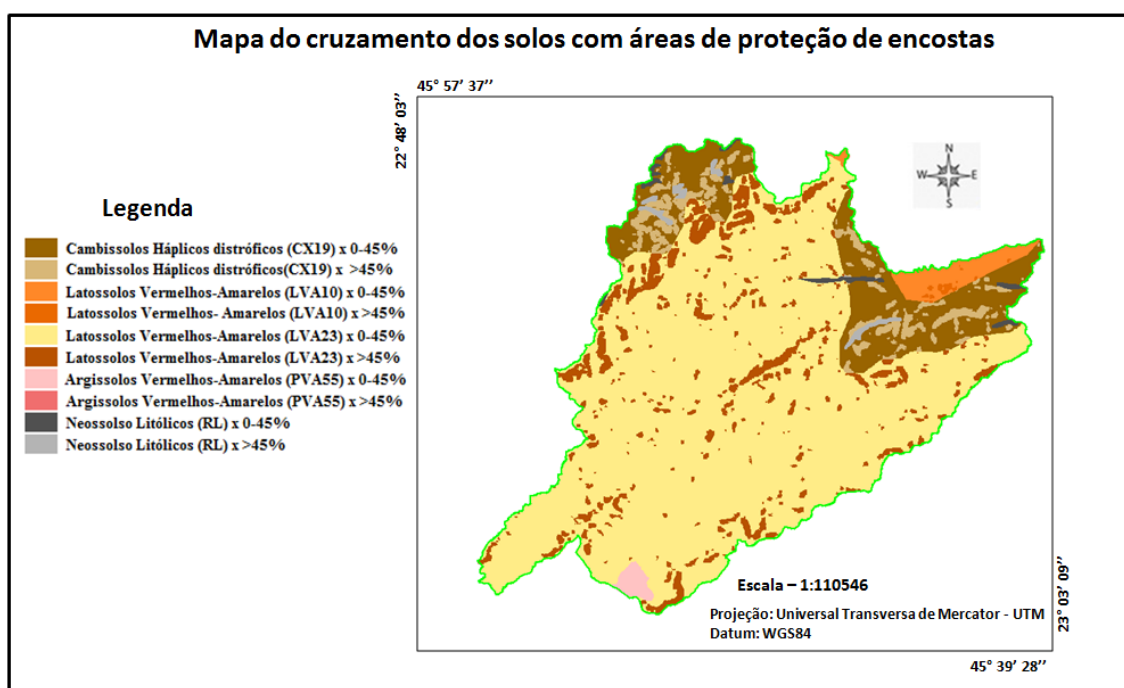
Figura 36: Distribuição das unidades de solos de acordo com a unidade de conservação das encostas.
