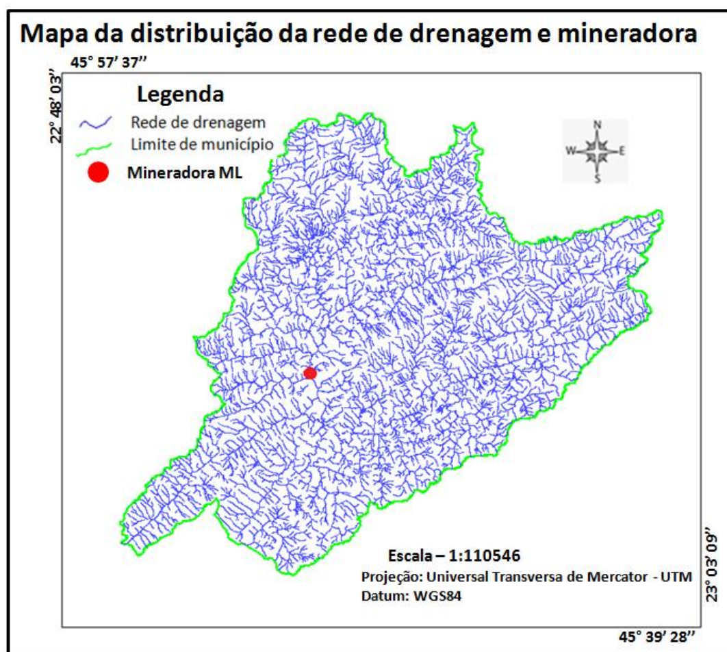
Figura 11: Mapa da distribuição da rede de drenagem e mineradoras de Monteiro Lobato.
