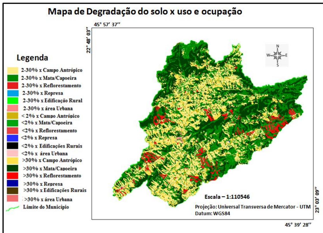
Figura 37: Distribuição do uso e ocupação do solo nas categorias de risco de acordo com Carvalho e Pinto (2009) para o município de Monteiro Lobato.
